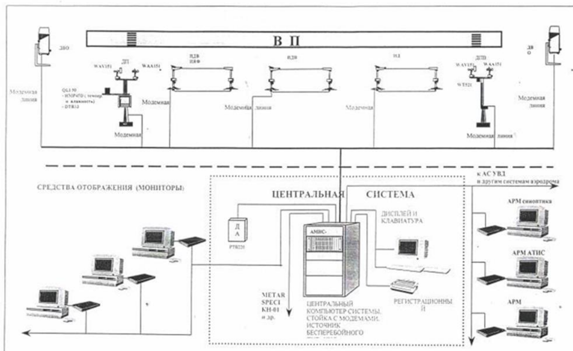
Рисунок 3 - Схема расположения АМИС-РФ
