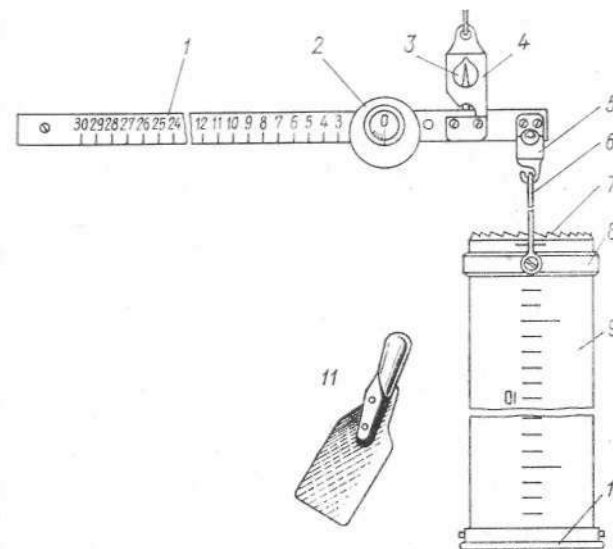
Рис. 1.9.2. Снегомер весовой ВС-43.
