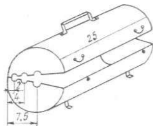
Рис. 1.10.2. Ванна для оттаивания гололедного отложения.
