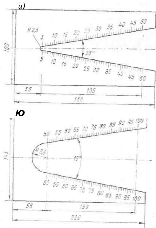
Рис. 1.10.5. Гололедный шаблон для измерения отложений.
