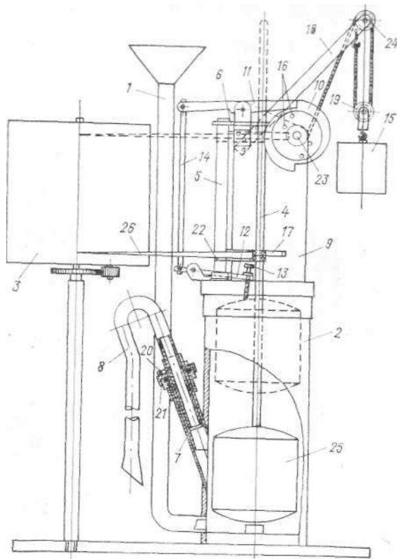
Рис. 1.8.5. Механизм принудительного слива плевниографа.
