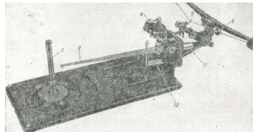
Рис. 1.5.2. Гигрограф М-21ЛС.
