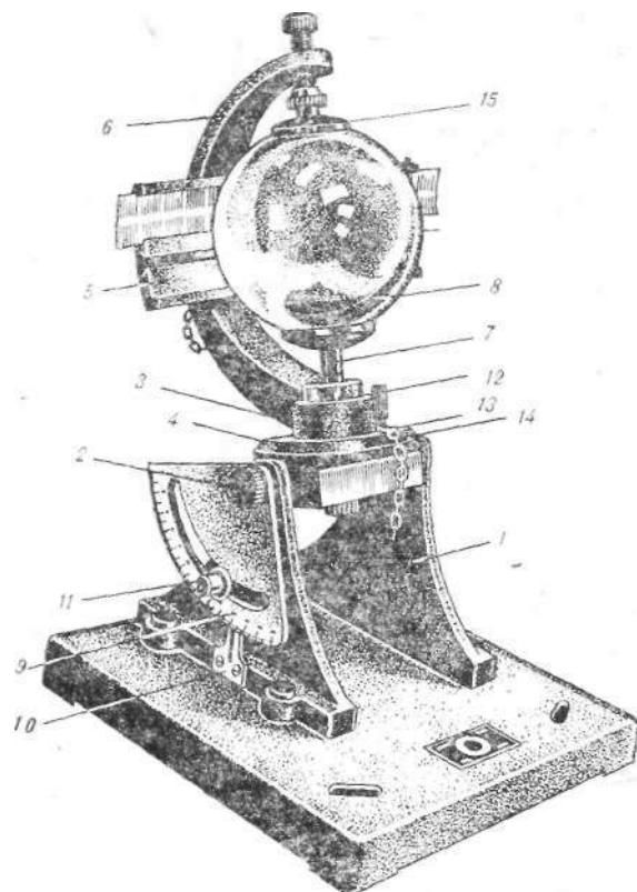
Рис. 1.6.1. Гелиограф универсальный модели ГУ-1.
