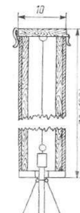
Рис. 1.7.8. Деревянный футляр для защиты вытяжных почвенно-глубинных термометров при высоком снежном покрове (разрез).
