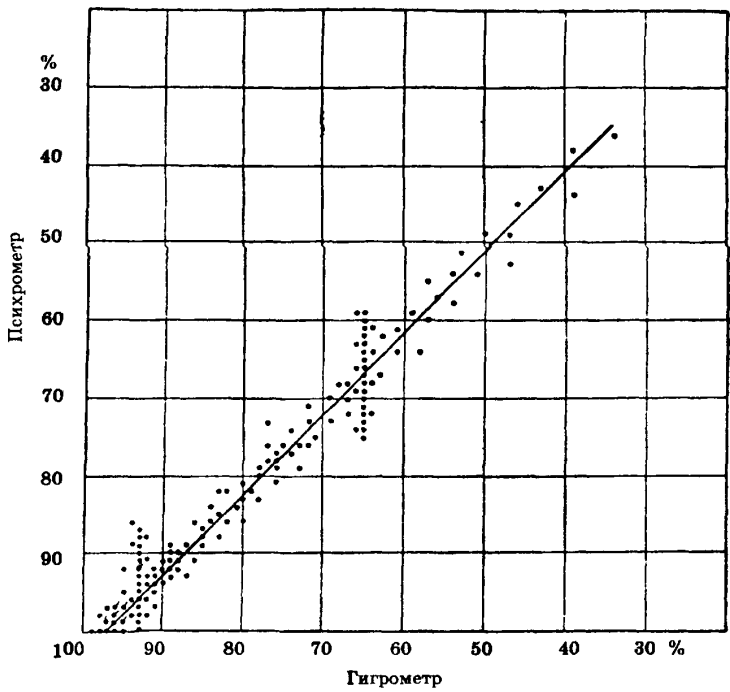
Рисунок 2 — График сравнения гигрометра и психрометра (ТМ-9) при трении или примерзании стрелки гигрометра
